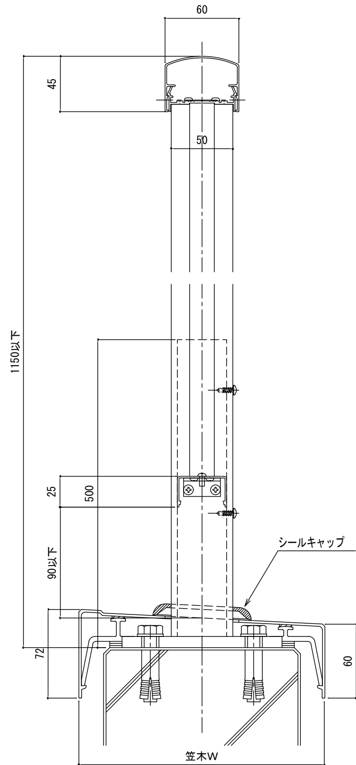
手すり断面図 (S : 1 / 3)
