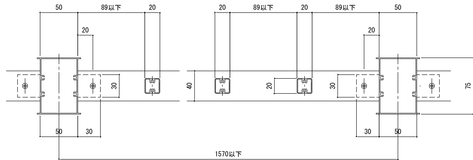
手すりユニット横断面図 (S : 1 / 3)
