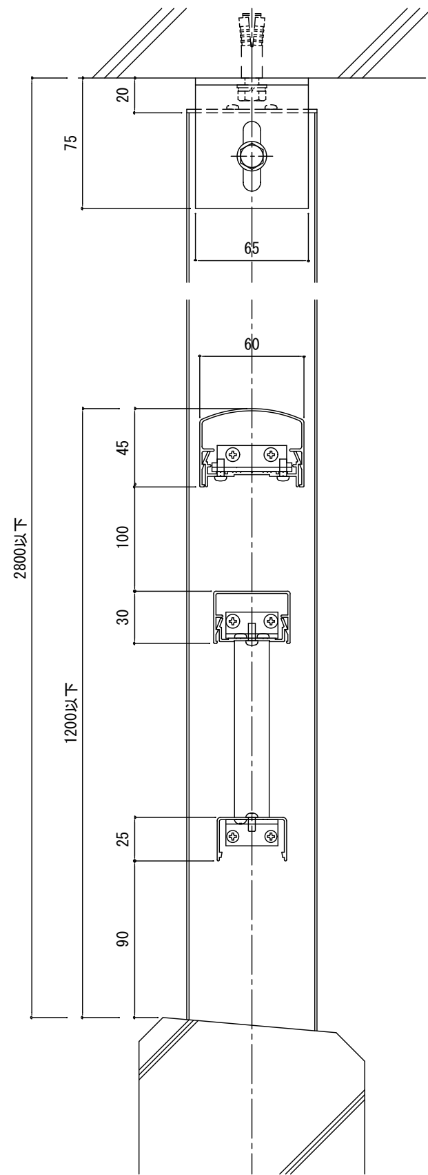
手すり断面図 (S : 1 / 3)
