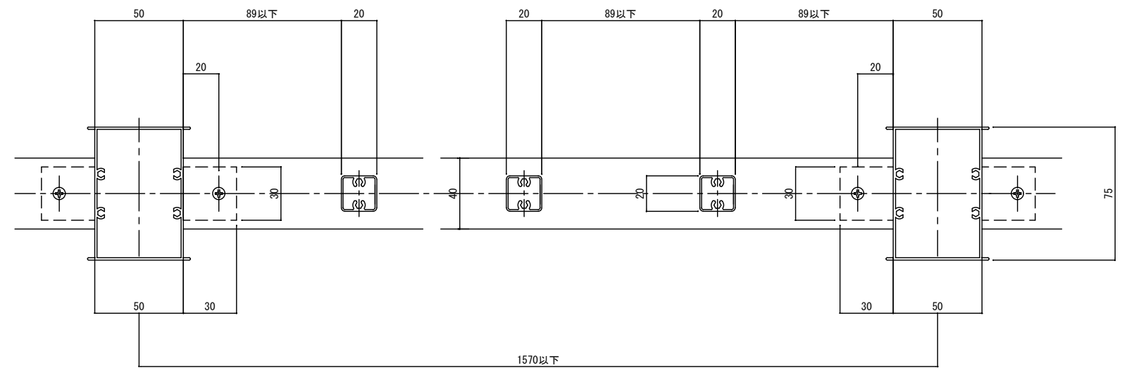
手すりユニット横断面図 (S : 1 / 3)
