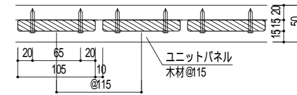
B部詳細図 (1/5)
