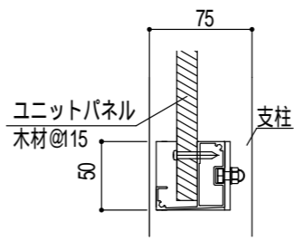
E部詳細図 (1/5)
