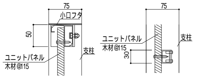
C部詳細図 (1/5)
