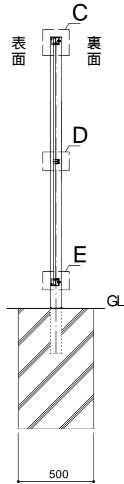
断面図 (1/25)
