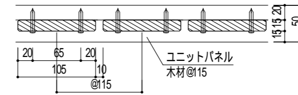
部詳細図 (1/5)
