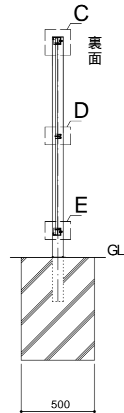
断面図 (1/25)
