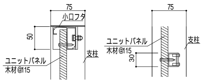
部詳細図 (1/5)
