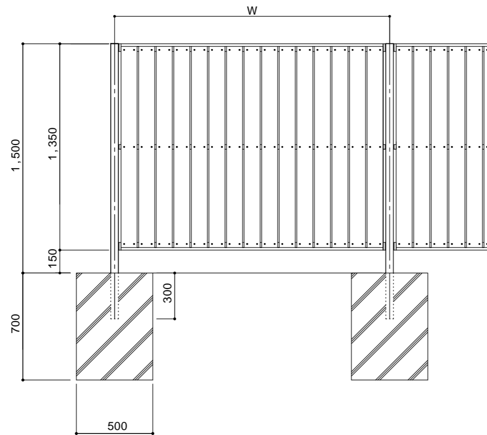
立面図 (1/25)
