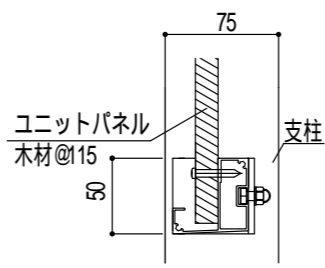
部詳細図 (1/5)
