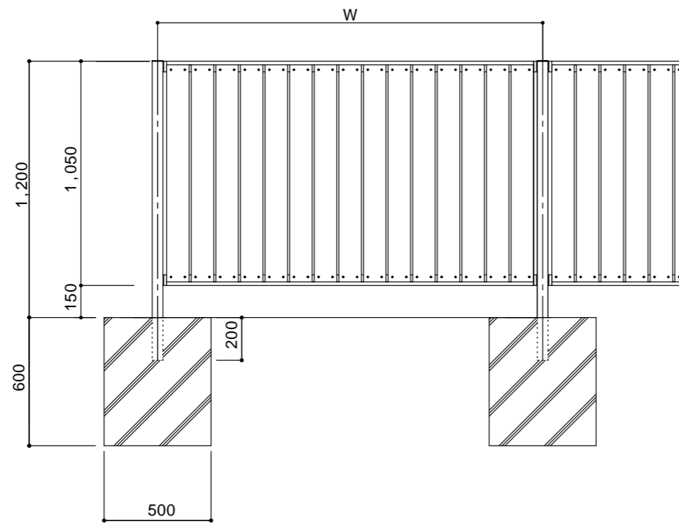
立面図 (1/25)
