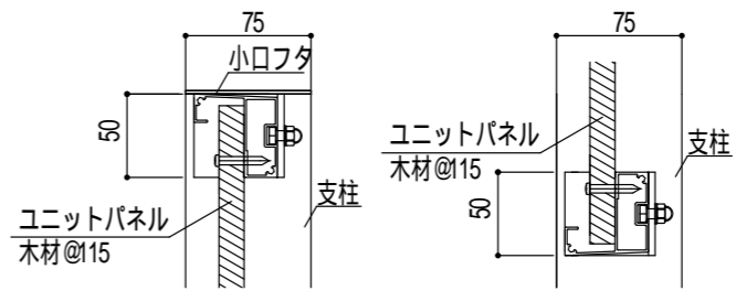
C部詳細図 (1/5)
