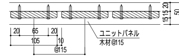
B部詳細図 (1/5)
