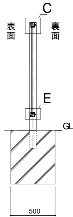
断面図 (1/25)
